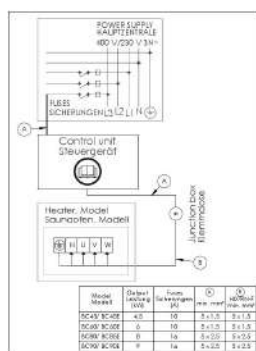
3-phase electrical connections of control unit C150 and BC-E heater 3-phasiger Elektronenschlüssel des Steuergeräts C150 und des Saunaofens BC-E
