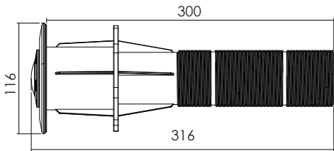
Conduits
